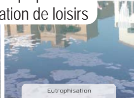
Eutrophisation
