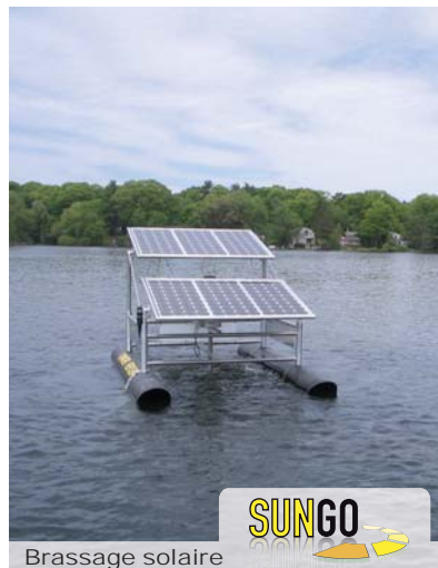
Brassage solaire
