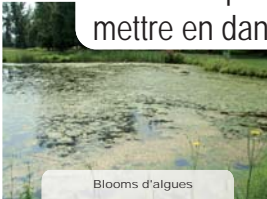
Blooms d'algues
